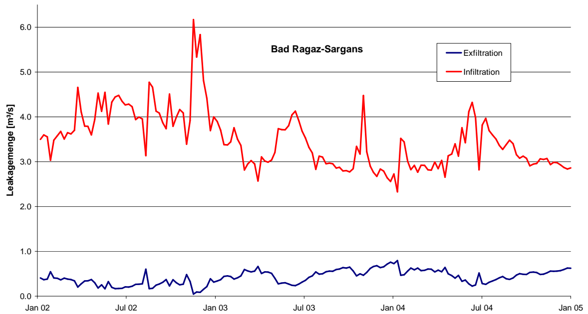
Abbildung 21 Zu- und Wegflüsse der Bäche oberhalb Eilhorn bis Landquart, links des Rheins
