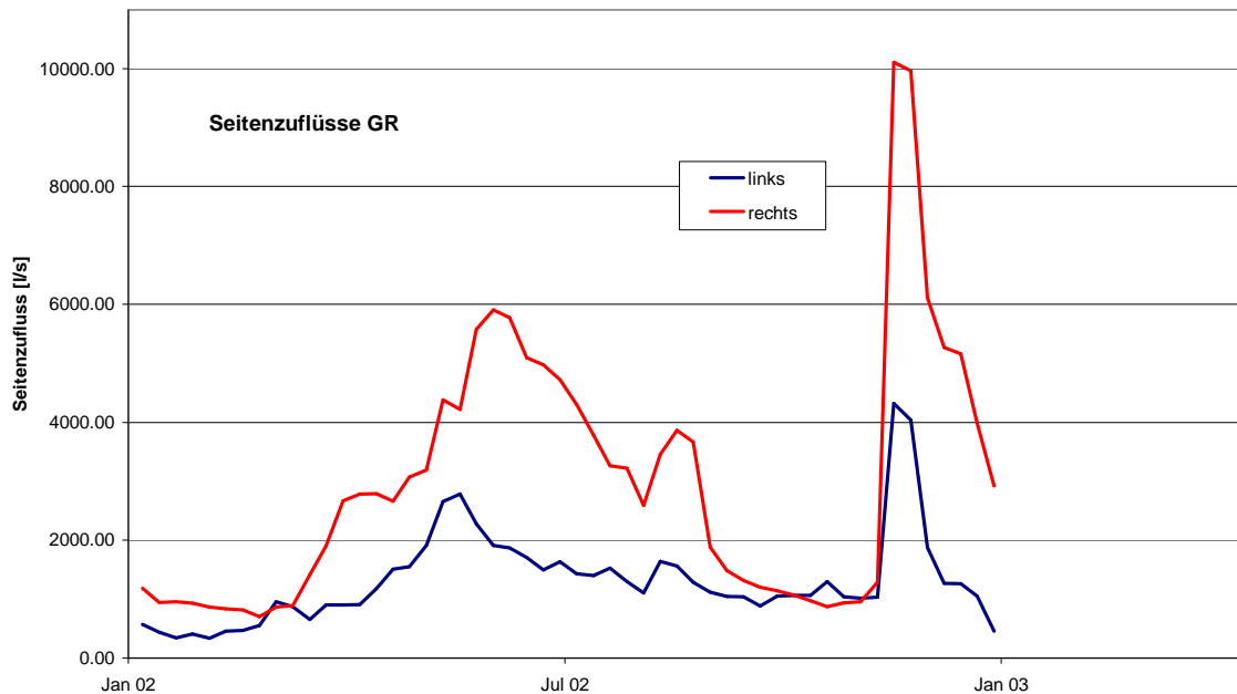
Abbildung 24 Seitenzuflüsse Kanton Graubünden. Linke Talseite von Reichenau bis Landquart, rechte Talseite von Reichenau bis Ellhorn
